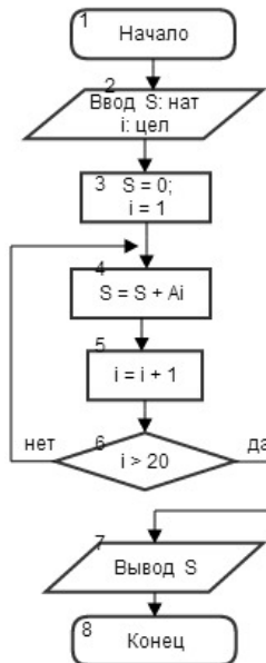
Рисунок 3 – Блок схема решения задачи 2
